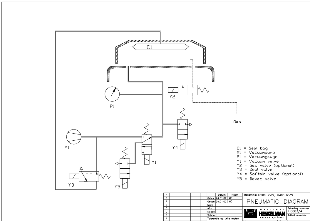
Pneumatisch schema H300RVS & H400RVS
