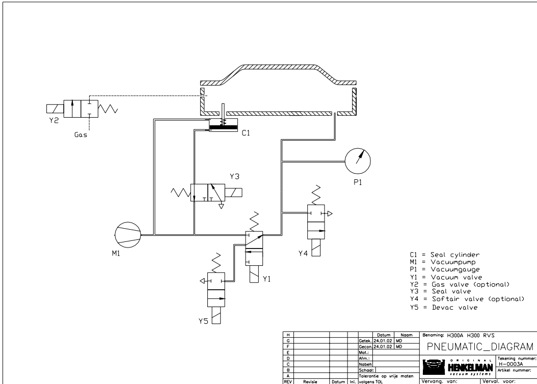
Pneumatisch schema H300A & H300
